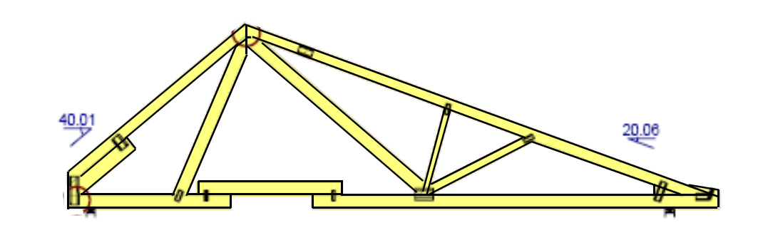
FACKVERK SPECIAL
