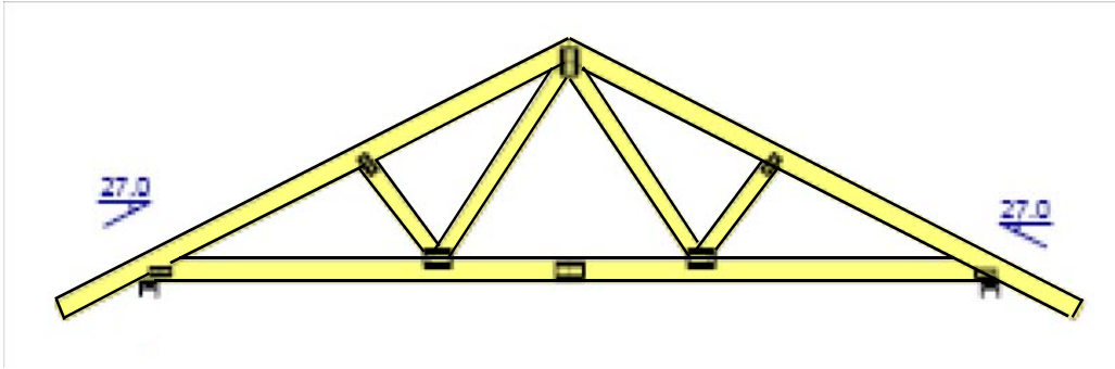
FACKVERK STANDARD
